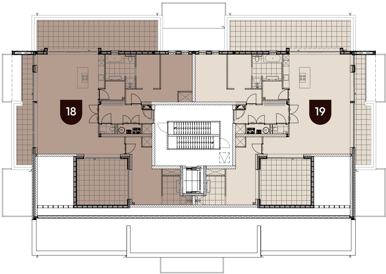
Derde verdieping
